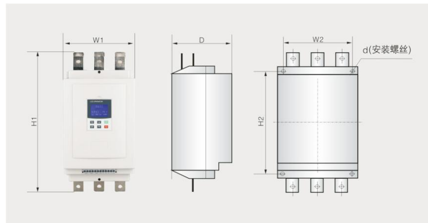
②75KW~600KW (图3.1.2)
