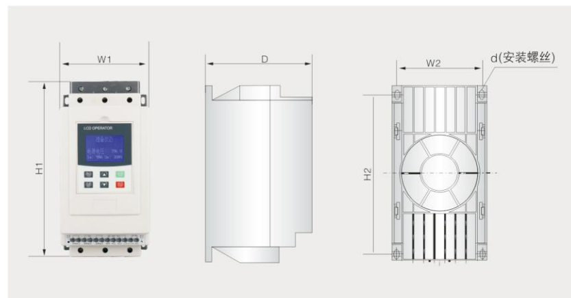
①11KW~75KW (图3.1.1)
